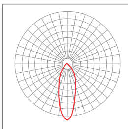
Ángulo de haz 38°
