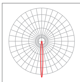
Ángulo de haz 12°
